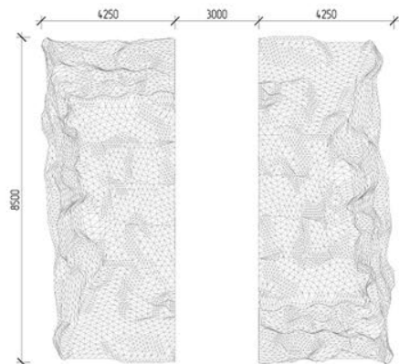
Вид сверху М 1:100
