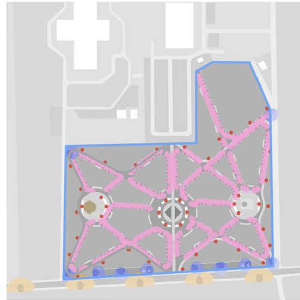
План освещения М 1:800
